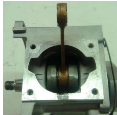
Carter y biela
